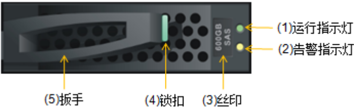
图3-27 3.5 英寸磁盘模块前面板
