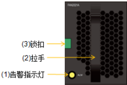
图3-17 DSU2625 风扇模块正视图
