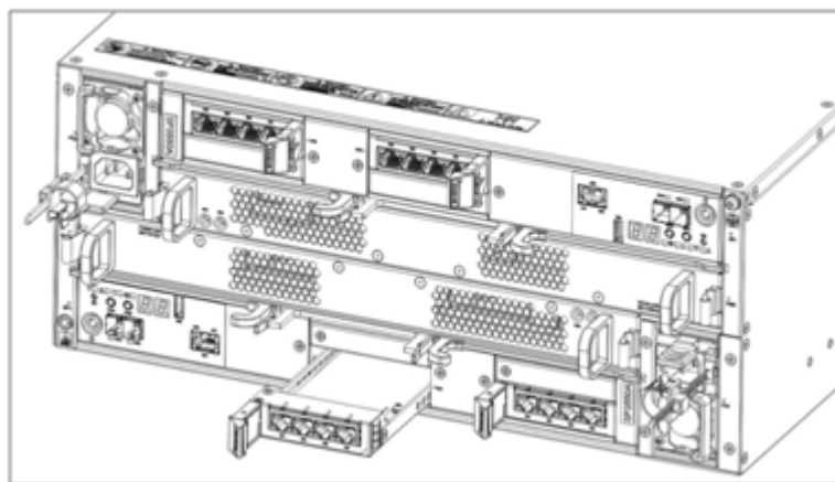
图6-8 安装/拆卸 IO 插卡示意图
