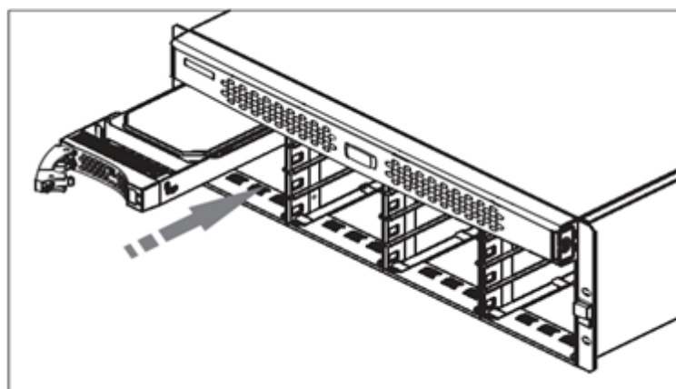
图6-21 安装 3.5 英寸磁盘模块 A 示意图（二）
