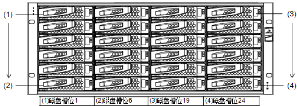
图6-23 DSU2624 磁盘槽位编号示意图
