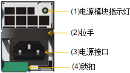
图3-7 MS3000G2-FT（16 盘位）SPU 电源模块正视图
