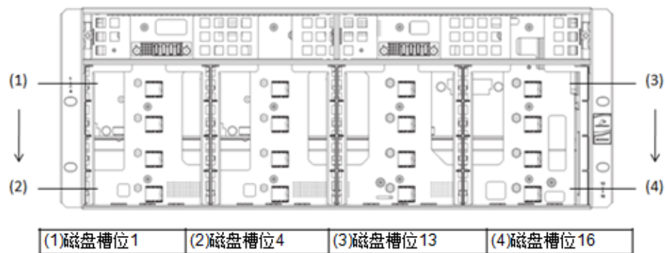
图6-19 MS3000G2-FT（16 盘位）SPU 磁盘槽位编号示意图
