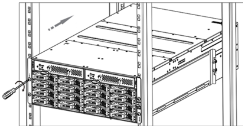
图4-13 安装 SPU 示意图
