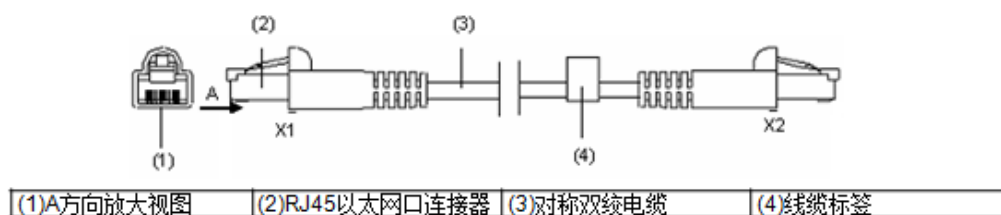
图4-38 GE 线缆示意图
