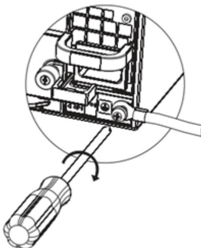
图4-26 安装接地线示意图
