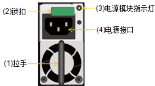
图3-13 MS3000G2-FT（24 盘位）SPU 电源模块正视图
