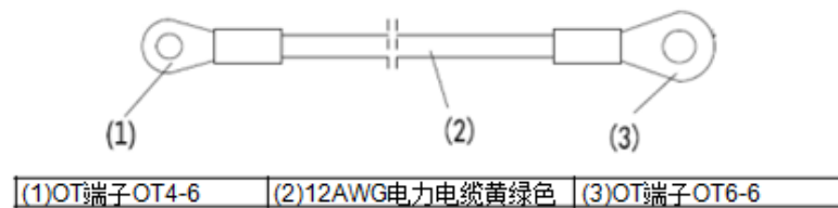
图4-24 接地线示意图
