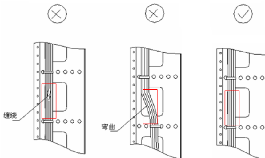
图4-20 线缆捆扎示意图（一）
