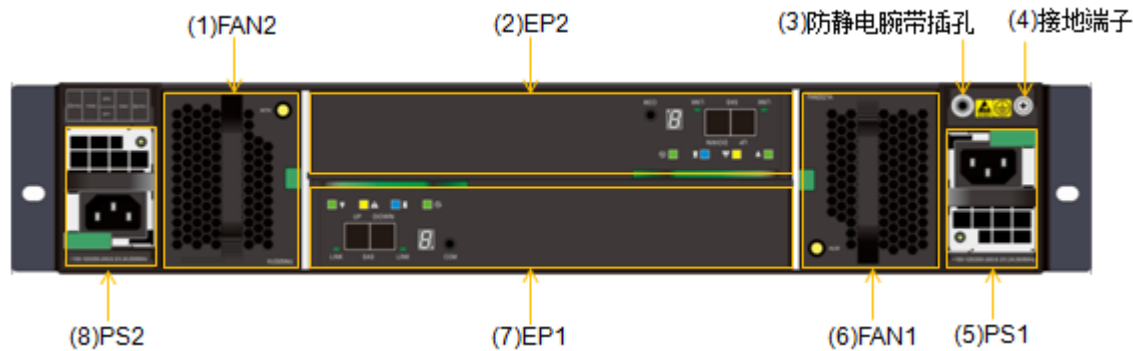
图3-15 DSU2625 后正视图
