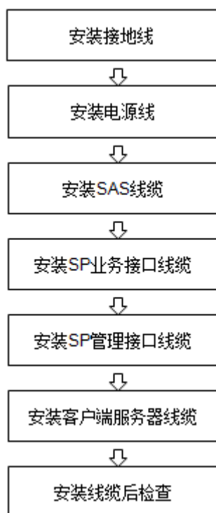
图4-23 线缆安装流程示意图
