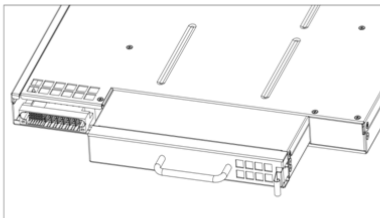
图6-7 安装/拆卸电池模块示意图
