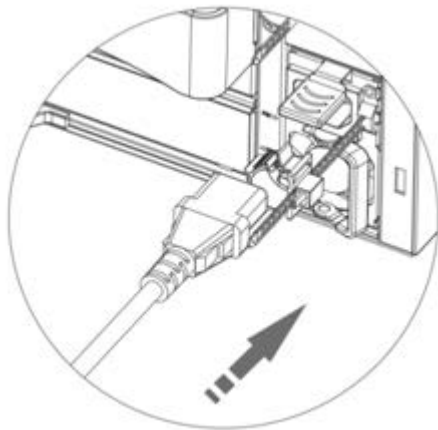
图4-29 安装电源线示意图（二）
