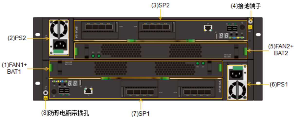
图3-9 MS3000G2-FT（24 盘位）SPU 后正视图
