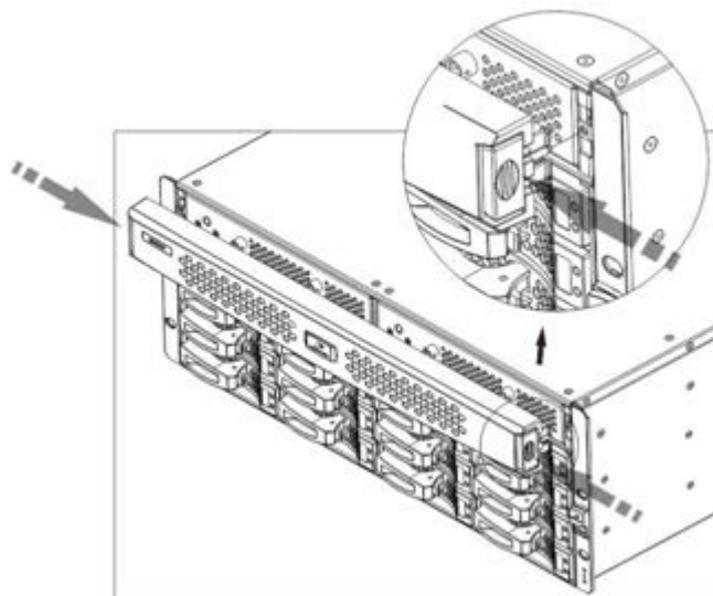
图4-16 安装 MS3000G2-FT（16 盘位）SPU 面板示意图
