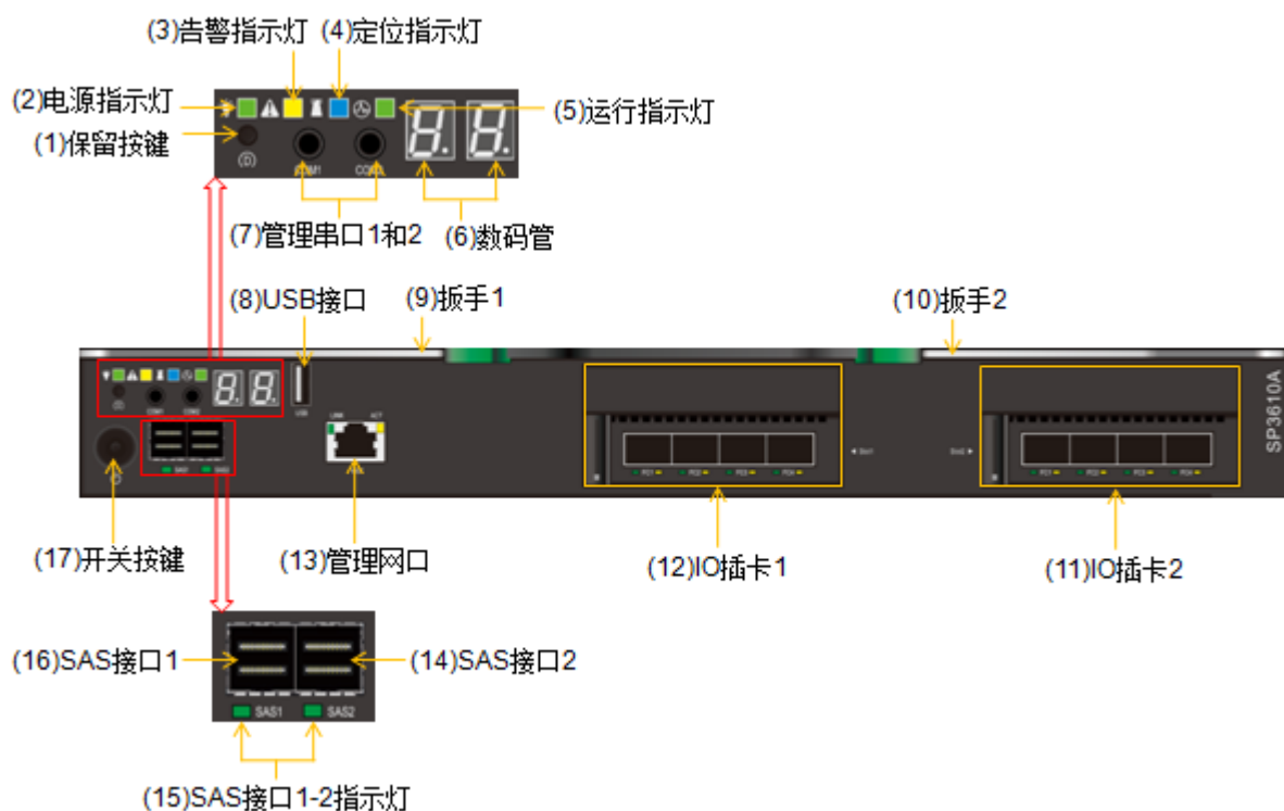
图3-10 MS3000G2-FT（24 盘位）SP 正视图
