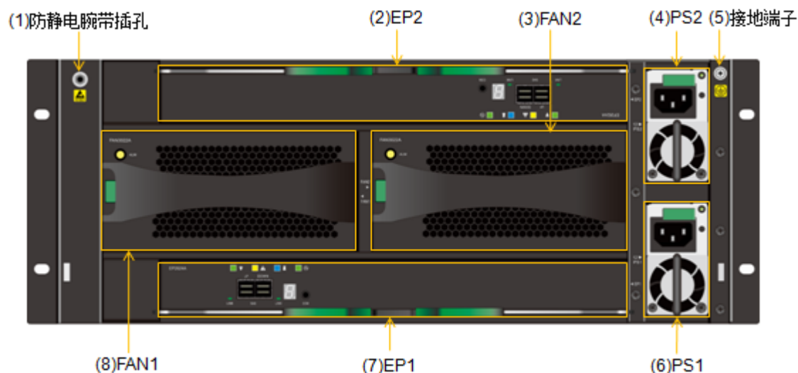
图3-20 DSU2624 后正视图
