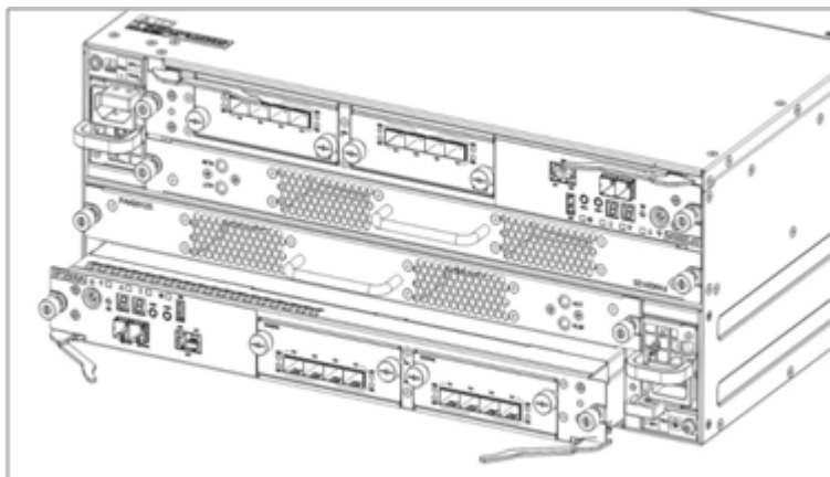
图6-2 安装/拆卸 MS3000G2-FT（16 盘位）SP 示意图
