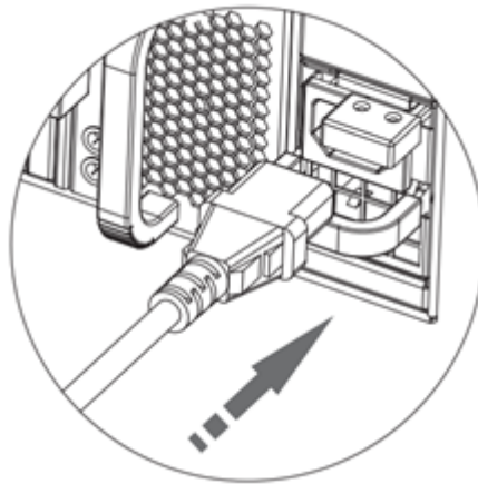
图4-28 安装电源线示意图（一）
