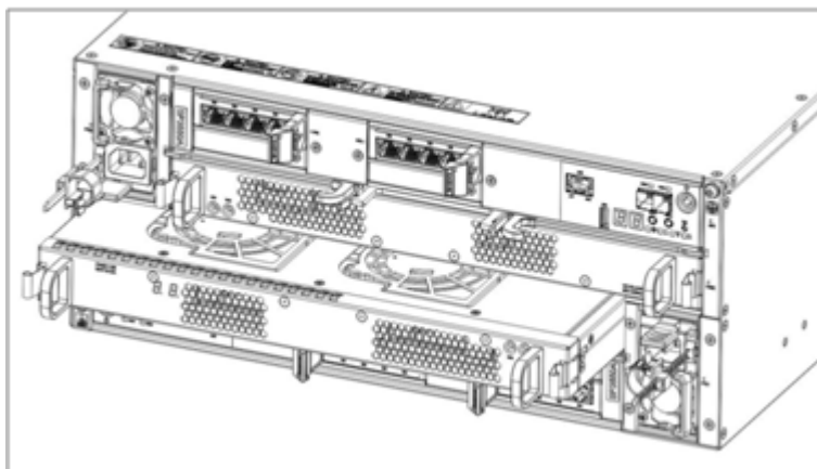
图6-6 安装/拆卸 MS3000G2-FT (24 盘位) SPU 风扇模块+电池模块示意图
