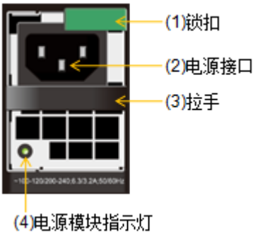
图3-18 DSU2625 电源模块正视图
