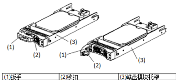
图6-18 3.5 英寸磁盘模块 A 示意图
