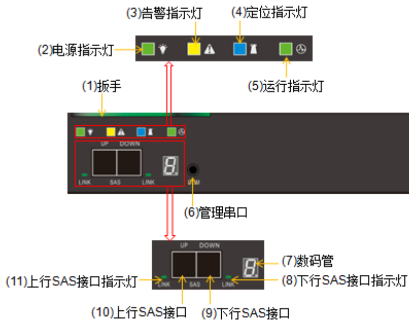
图3-16 DSU2625 的 EP 正视图
