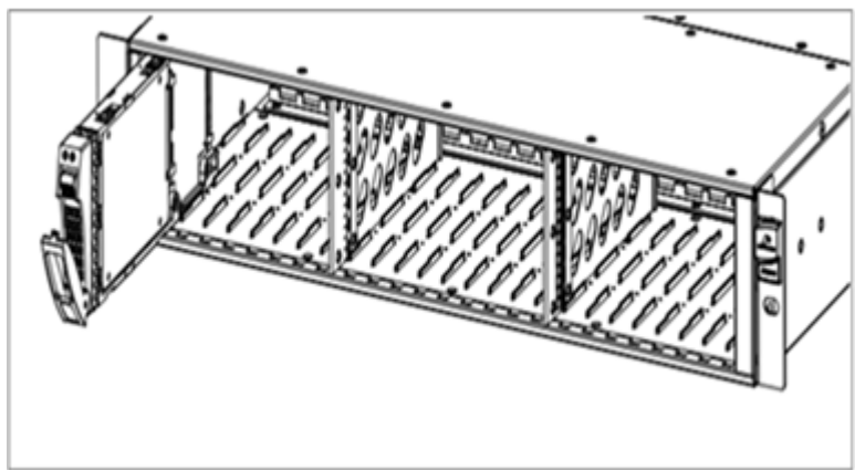
图6-17 安装 2.5 英寸磁盘模块示意图（二）
