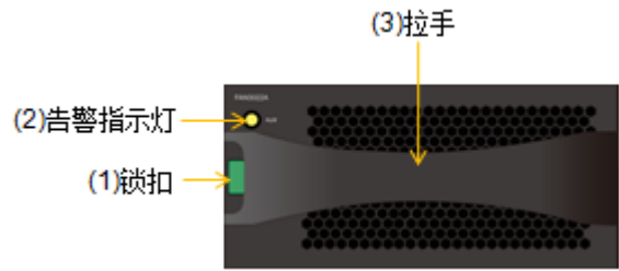
图3-22 DSU2624 风扇模块正视图
