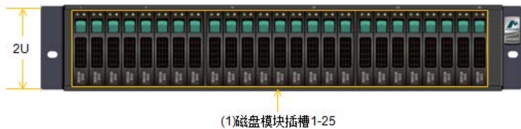
图3-14 DSU2625 前正视图
