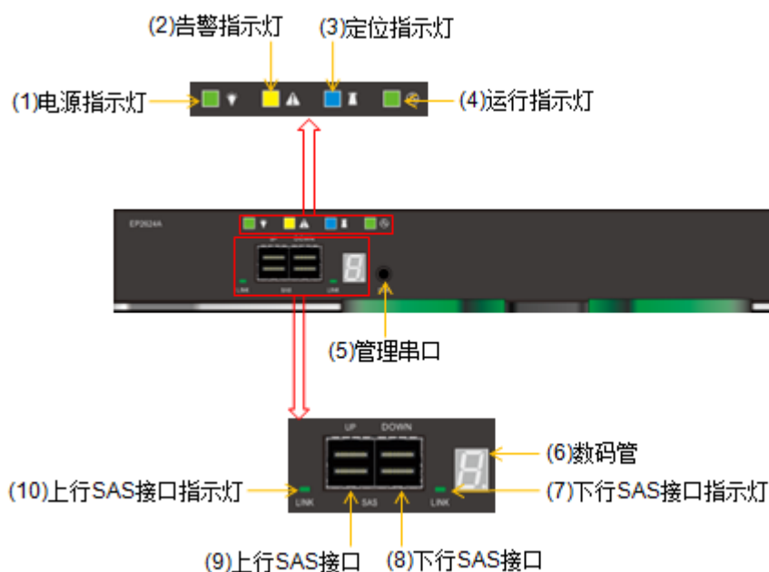
图3-21 DSU2624 的 EP 正视图
