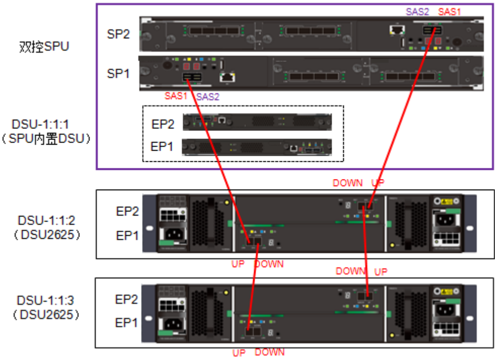
图4-35 SAS1 接口上 SAS 线缆安装示意图
