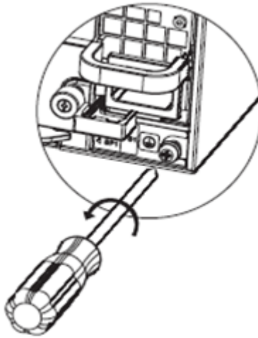
图4-25 松开设备接地端子的螺钉示意图
