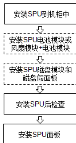
图4-12 SPU 安装流程示意图
