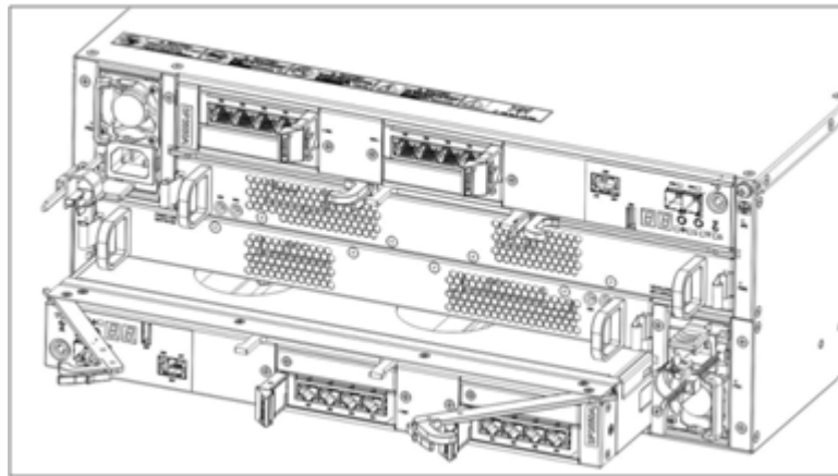
图6-3 安装/拆卸 MS3000G2-FT（24 盘位）SP 示意图
