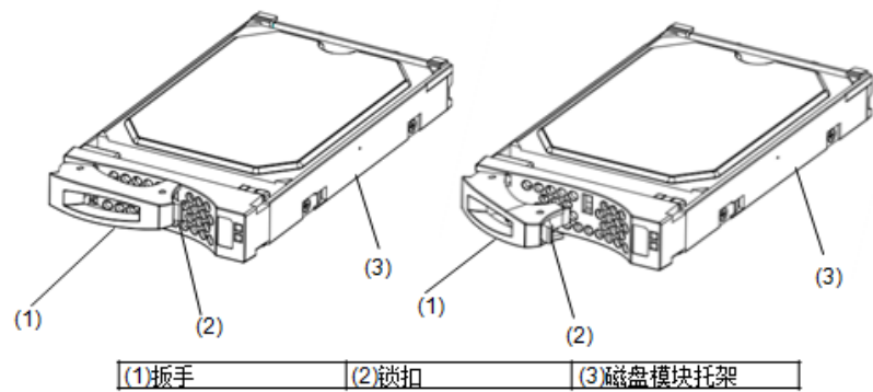
图6-22 3.5 英寸磁盘模块 B 示意图
