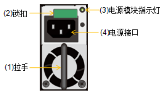
图3-23 DSU2624 电源模块正视图
