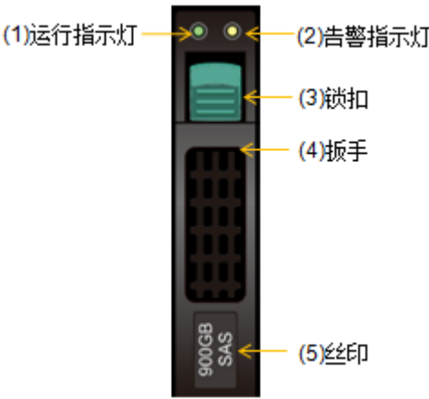
图3-24 2.5 英寸磁盘模块前面板
