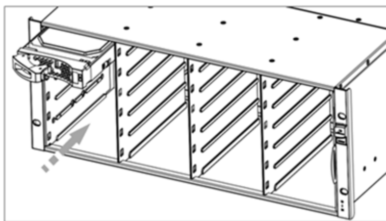
图6-25 安装 3.5 英寸磁盘模块 B 示意图（二）
