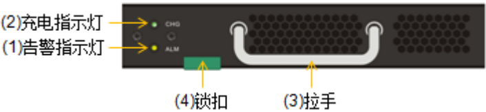
图3-6 MS3000G2-FT（16 盘位）SPU 电池模块正视图
