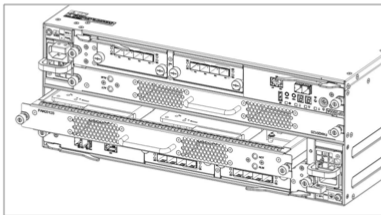
图6-4 安装/拆卸 MS3000G2-FT (16 盘位) SPU 风扇模块示意图
