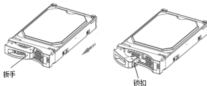
图6-24 安装 3.5 英寸磁盘模块 B 示意图（一）
