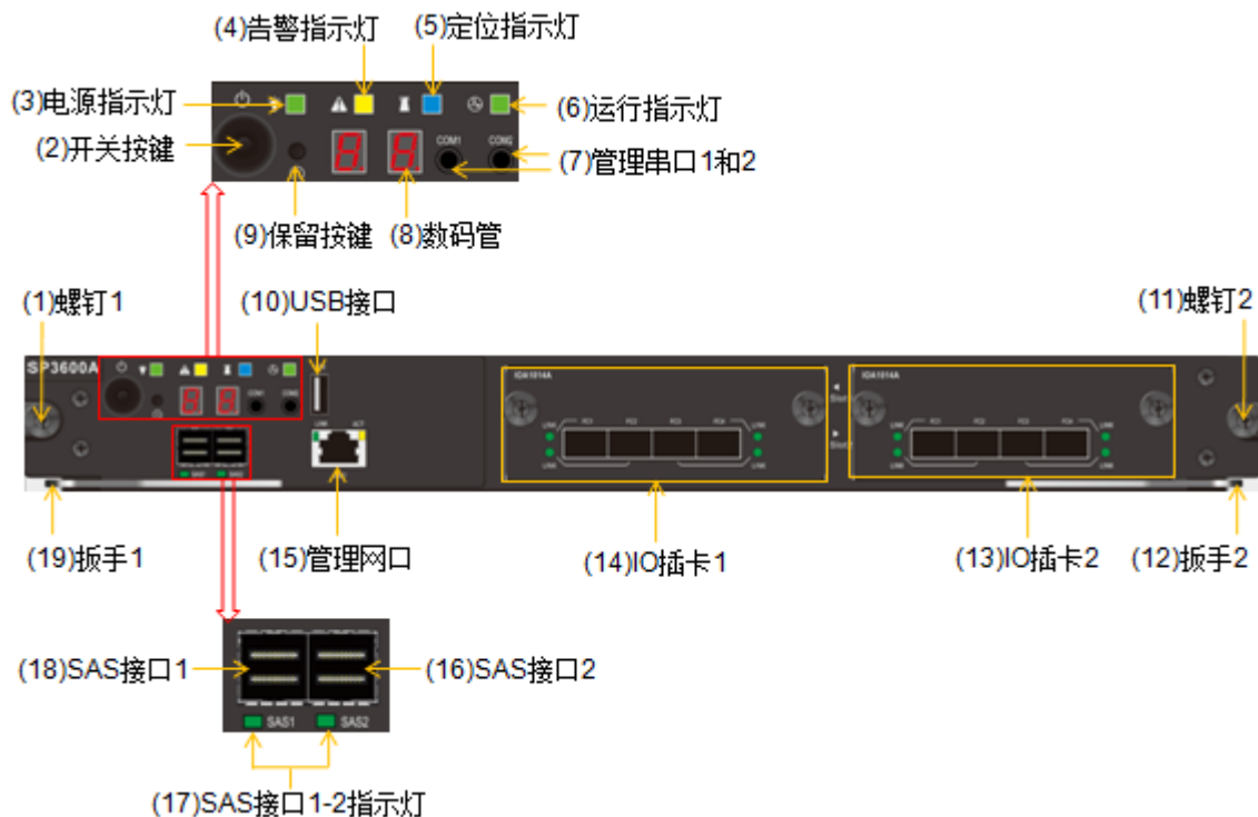
图3-4 MS3000G2-FT（16 盘位）SP 正视图
