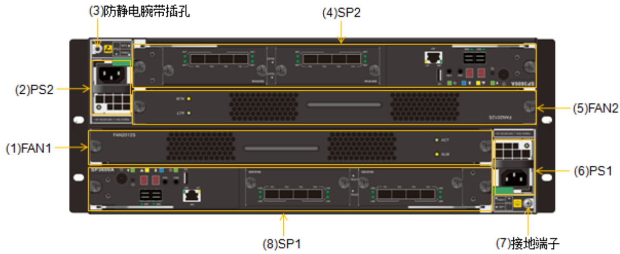
图3-3 MS3000G2-FT（16 盘位）SPU 后正视图
