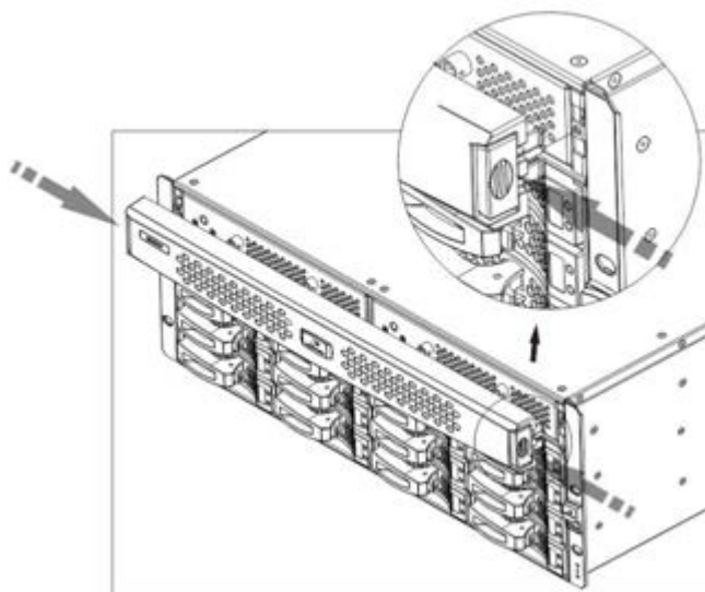
图6-1 安装/拆卸 MS3000G2-FT（16 盘位）SPU 面板示意图
