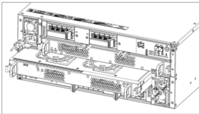
图4-15 安装 MS3000G2-FT（24 盘位）SPU 风扇模块+电池模块示意图
