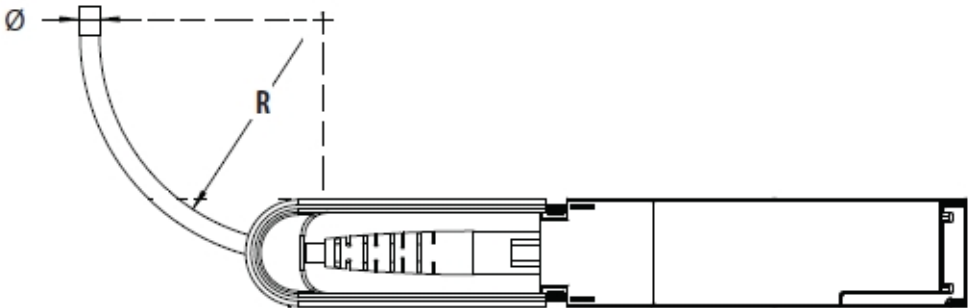
图4-34 AOC 光缆弯曲半径示意图
