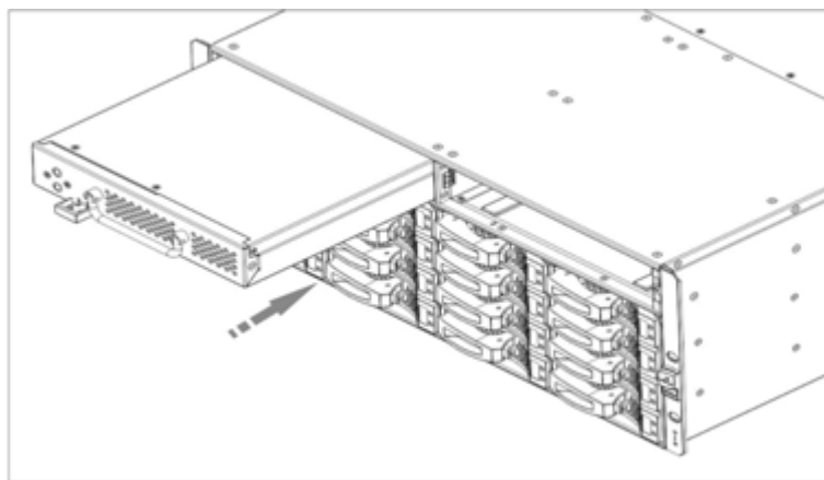
图4-14 安装 MS3000G2-FT（16 盘位）SPU 电池模块示意图
